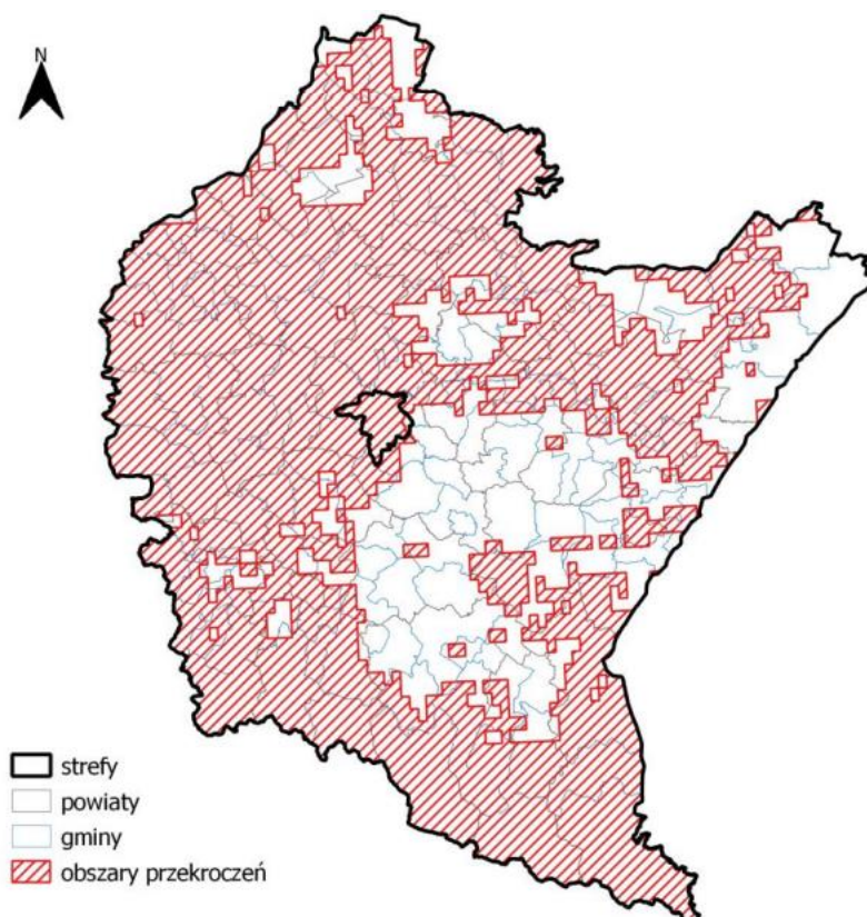
RYСУNEK 5. ZASIĘG OBSZARÓW PRZEKROCZEŃ POZIOMU CELU DŁUGOTERMINOWEGO OZONU DLA 8-GODZ. STĘŻENIA O 3 ZE WZGLĘDU NA OCHRONĘ ZDROWIA W WOJEWÓDZTWIE PODKARPACZYM W 2020 R.
